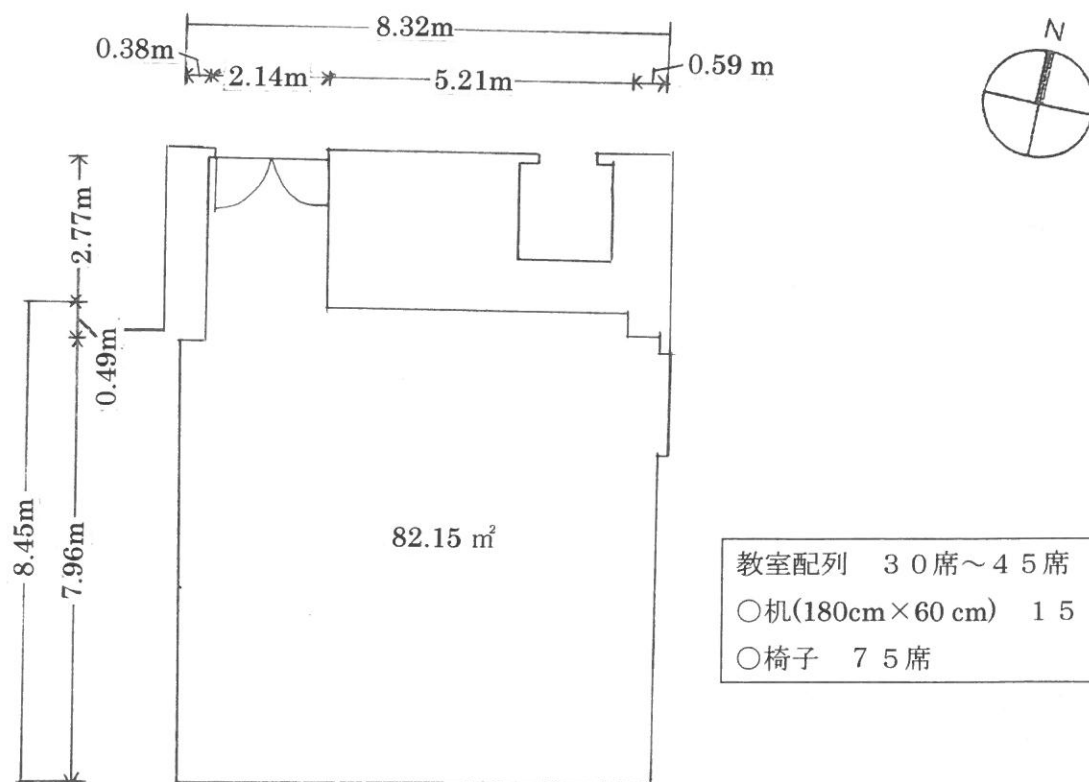
大西・アオイ記念館 立礼の間兼会議室平面図（2階）
